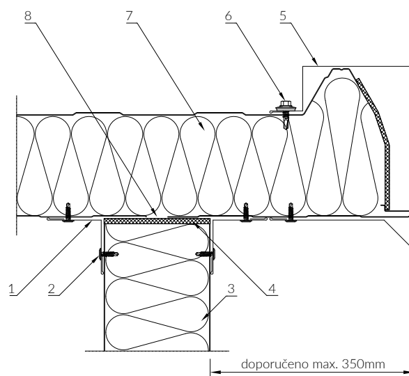
Výkres č. 52
