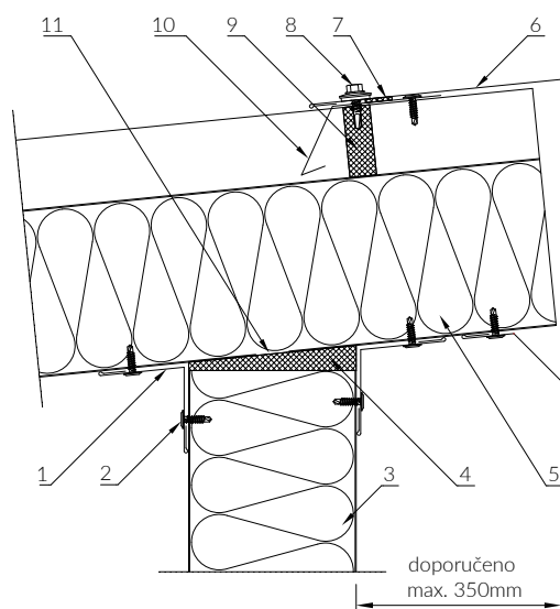
Výkres č. 50
