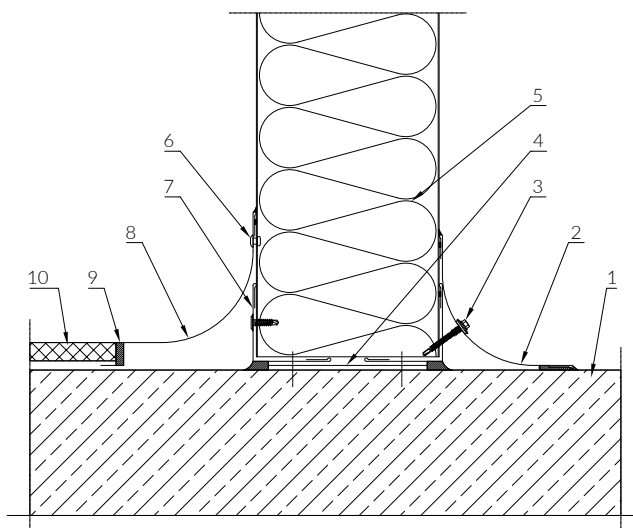
Výkres č. 31
