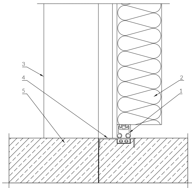
Výkres č. 43
