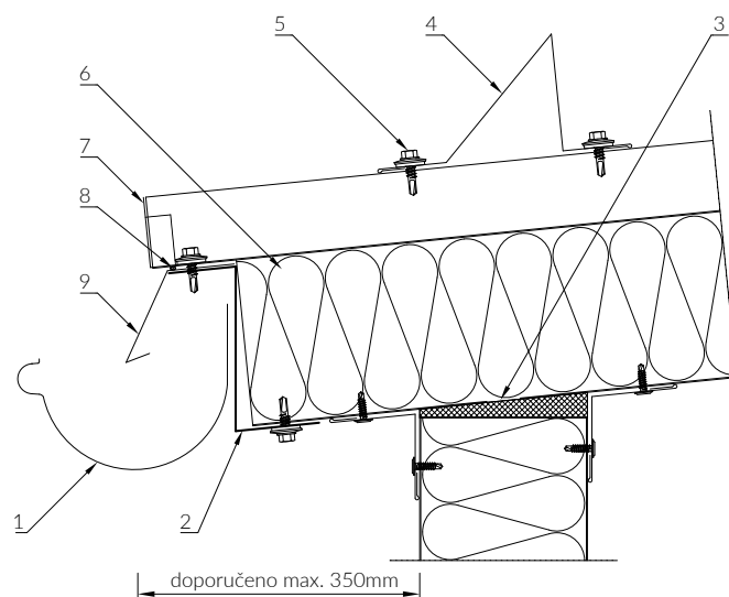
Výkres č. 45
