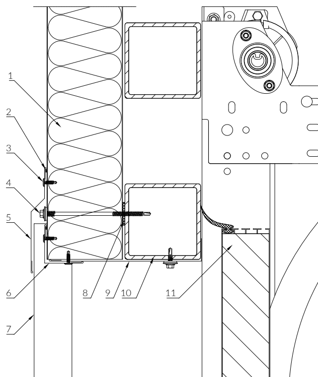
Výkres č. 15
