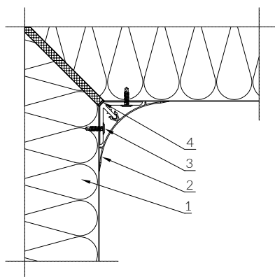
Výkres č. 35
