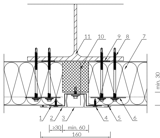
Výkres č. 11
