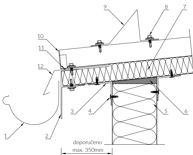
Výkres č. 48
