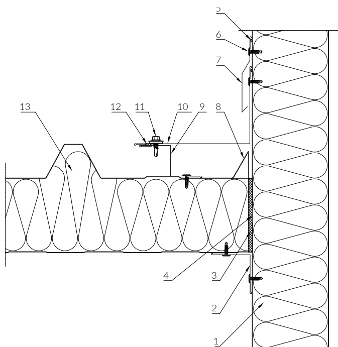
Výkres č. 55
