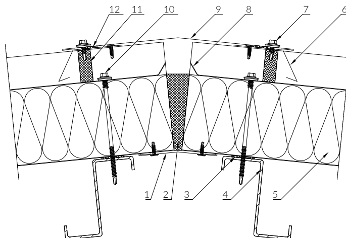
Výkres č. 44
