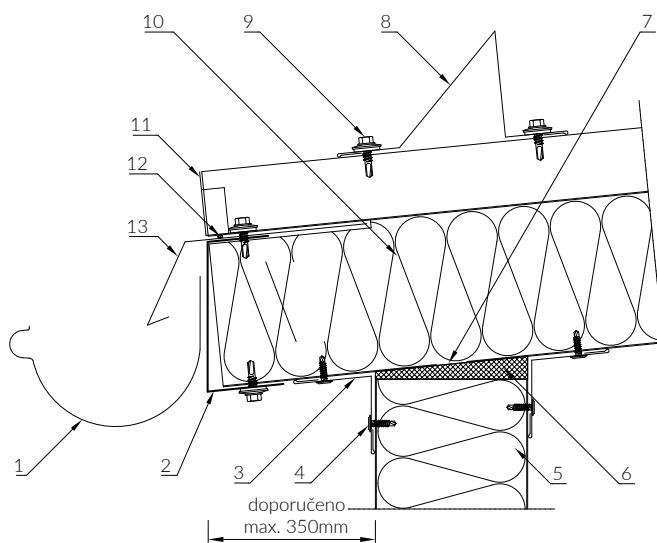
Výkres č. 47
