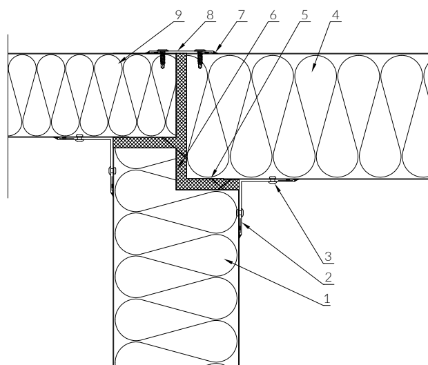
Výkres č. 38
