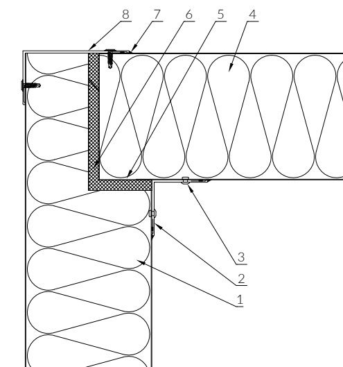
Výkres č. 37
