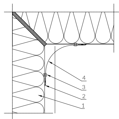
Výkres č. 34
