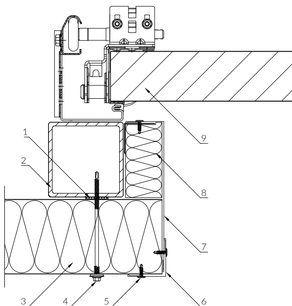
Výkres č. 18
