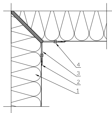
Výkres č. 33
