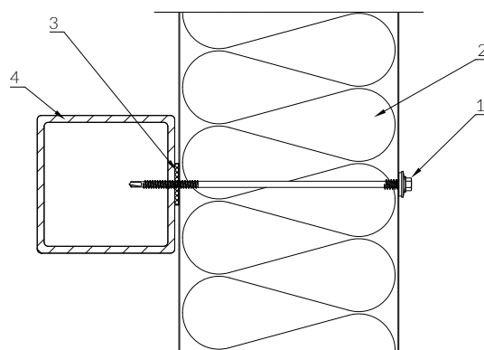
Výkres č. 23
