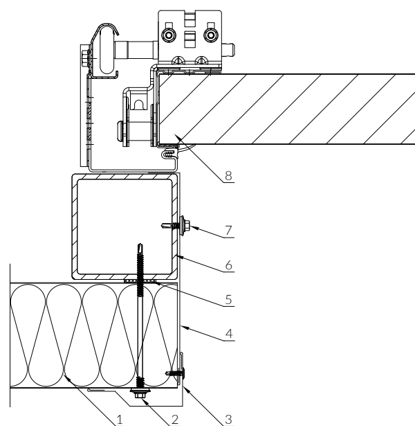
Výkres č. 16
