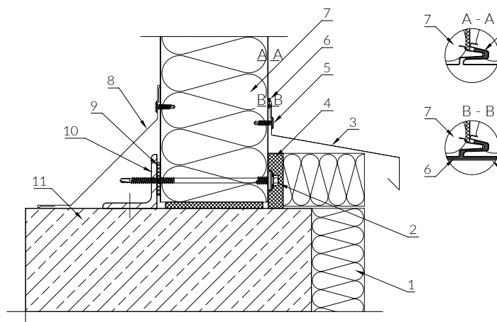
Výkres č. 3
