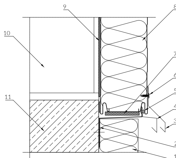
Výkres č. 5
