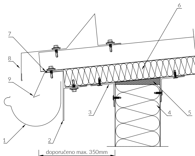
Výkres č. 46
